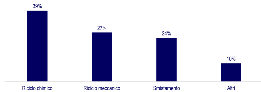
Figura 4.3. Brevetti per applicazione (valore percentuale sul totale riferito alla plastica). Fonte: elaborazione The European House - Ambrosetti su dati World Intellectual Property Organization ed European Patent Office, 2022.
